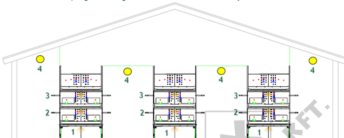
5. ábra: Az Unistart nevelőrendszer áttekintése. Az 1-es, 2-es és 3-as számok LED lámpák. Minden lámpa (1, 2,3,4) dimmerelő lámpa
