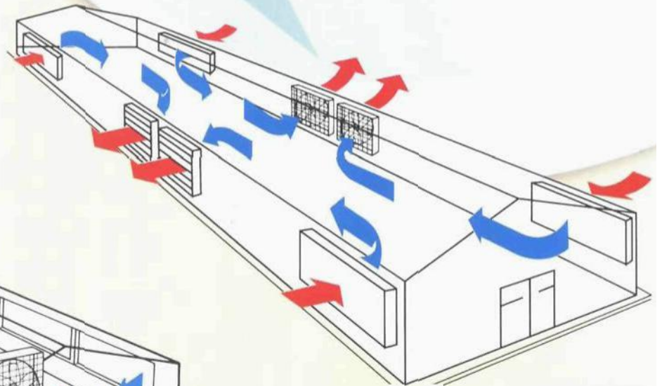
HOSSZIRÁNYÚ SZELL ZÉS LÉGVEZET FEJEKKEL (70 m-en túl)
