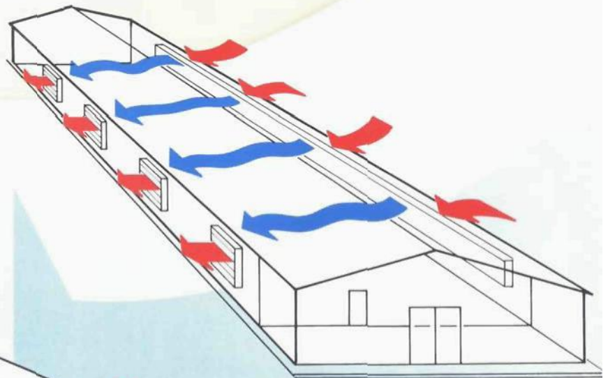
KERESZTIRÁNYÚ SZELL ZÉS
